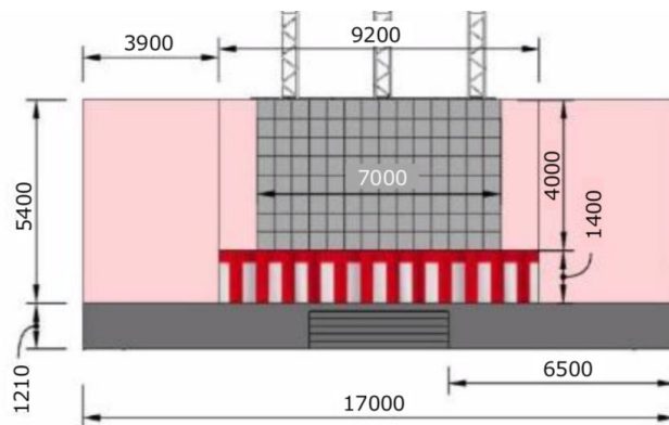
ステージ立面図
