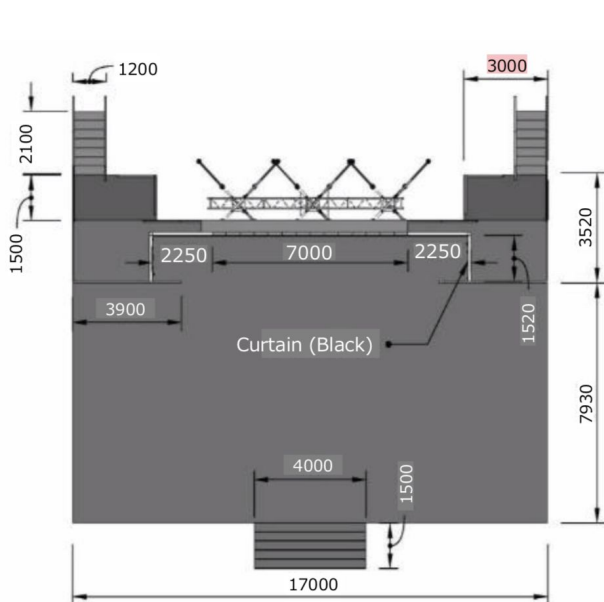
ステージ平面図
